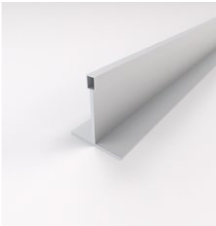
Sistema T.A. e T.N. per soffitto T.A. and T.N. system for ceiling
